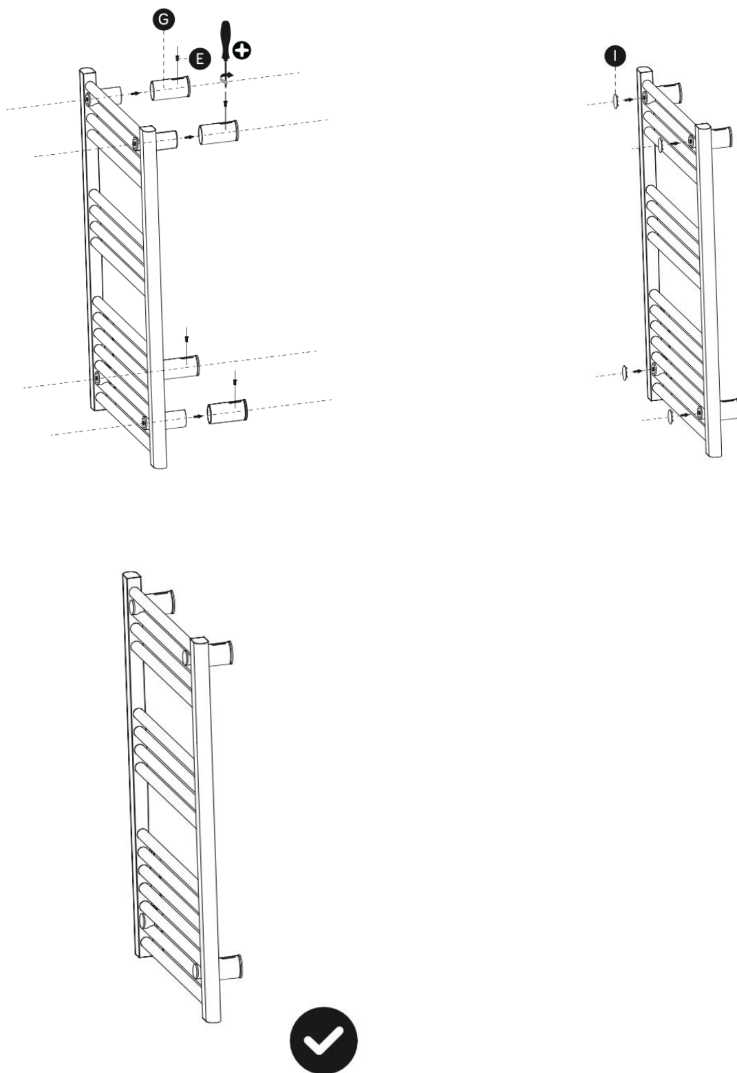
Рисунок 4. Монтаж техники
