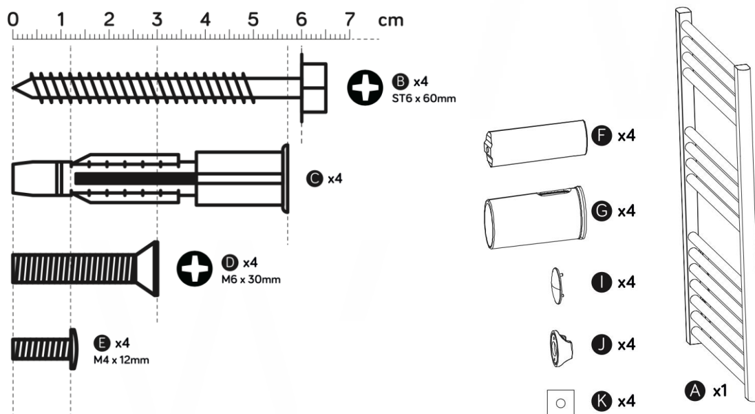
Рисунок 3. Крепежные элементы
