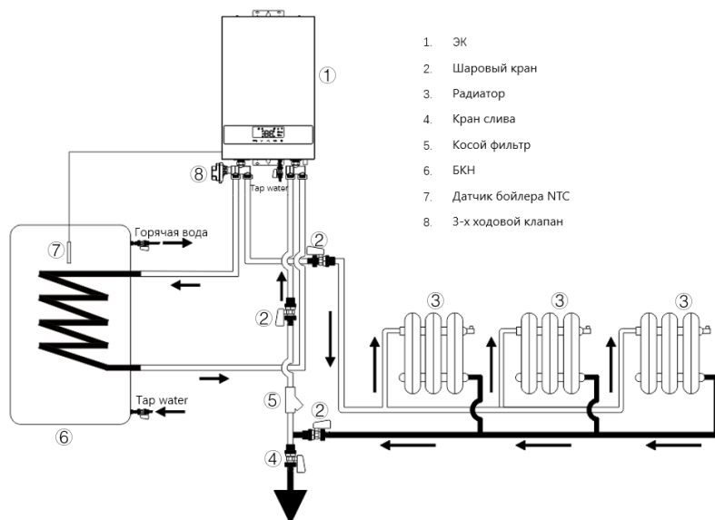
Рис. 19. Схема подключения «радиаторы + ЭК + БКН».
