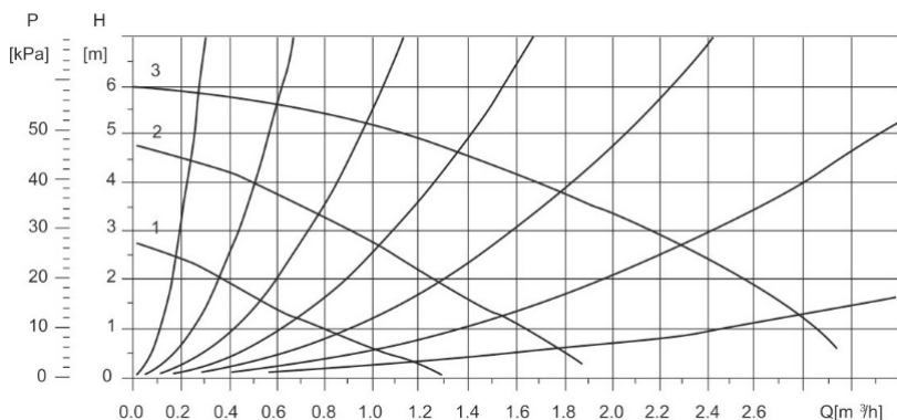
Рис. 22. Кривая характеристик давления насоса
