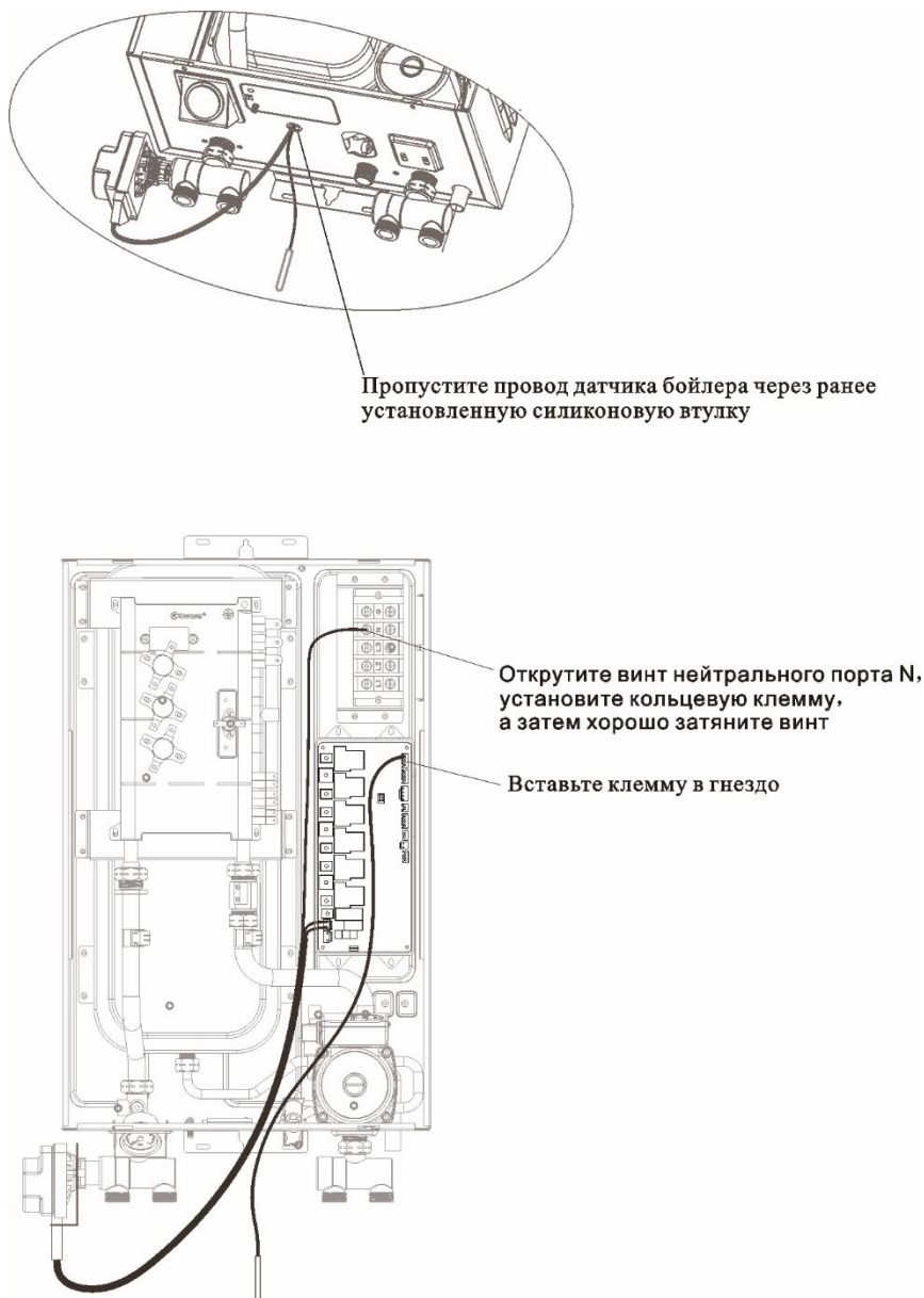
Рис. 18. Подключение датчика бойлера
