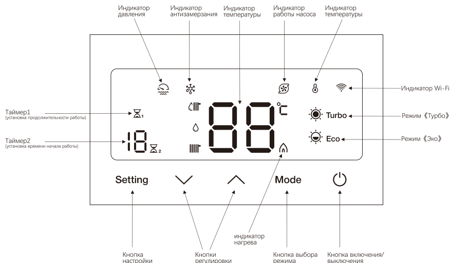
Рис. 3. Панель управления
