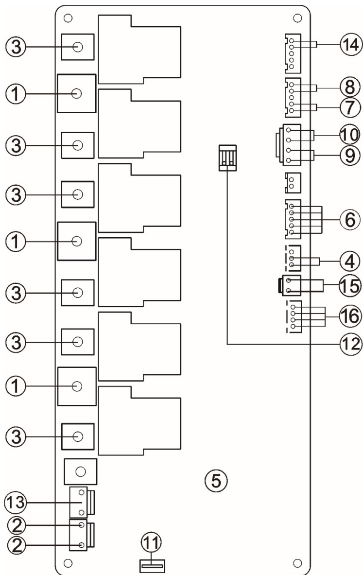
Рис. 24. Электрическая схема основной платы управления
