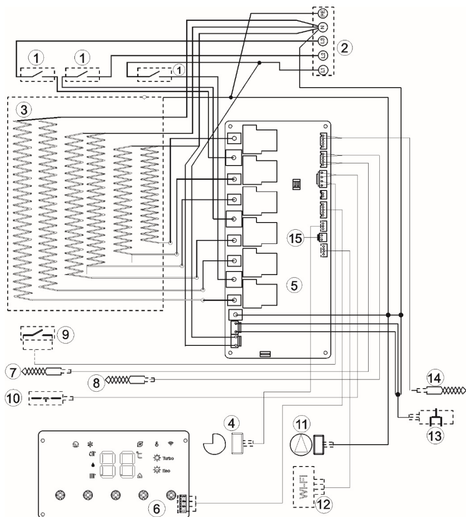
Рис. 23. Электрическая схема THERMEX Sonne 12 Wi-Fi
